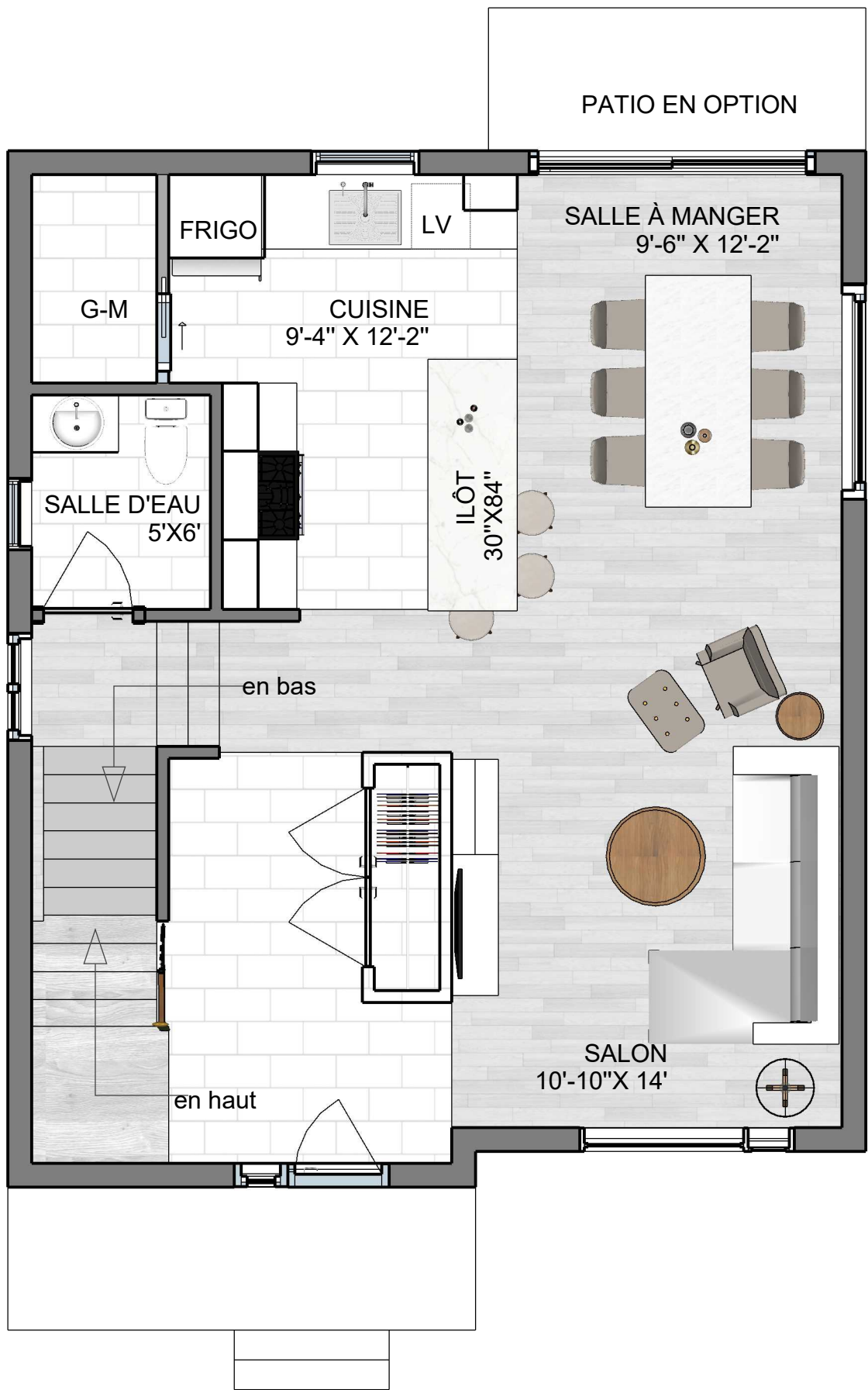
PLAN DU REZ-DE-CHAUSSEE MISTRAL
